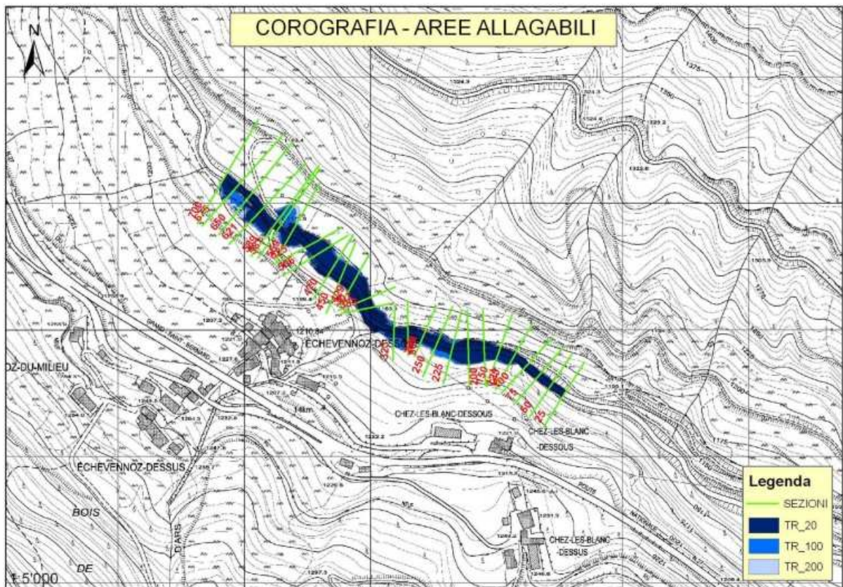
Tavola 2.1 – Confronto tra le aree allegate per i tempi di ritorno di 20, 100 e 200 anni risultanti dallo studio di approfondimento sul tratto dell’Artanavaz a cavallo della confluenza con il torrente Arsy (sotto) e la relativa perimetrazione dei vincoli per inondazione (Art. 36 l.r. 11/98) riportata nella cartografia prescrittiva degli ambiti inedificabili del Comune di Etroubles (sopra).
